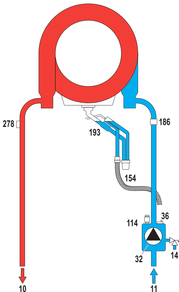
fig. 28 - Circuito hidráulico
