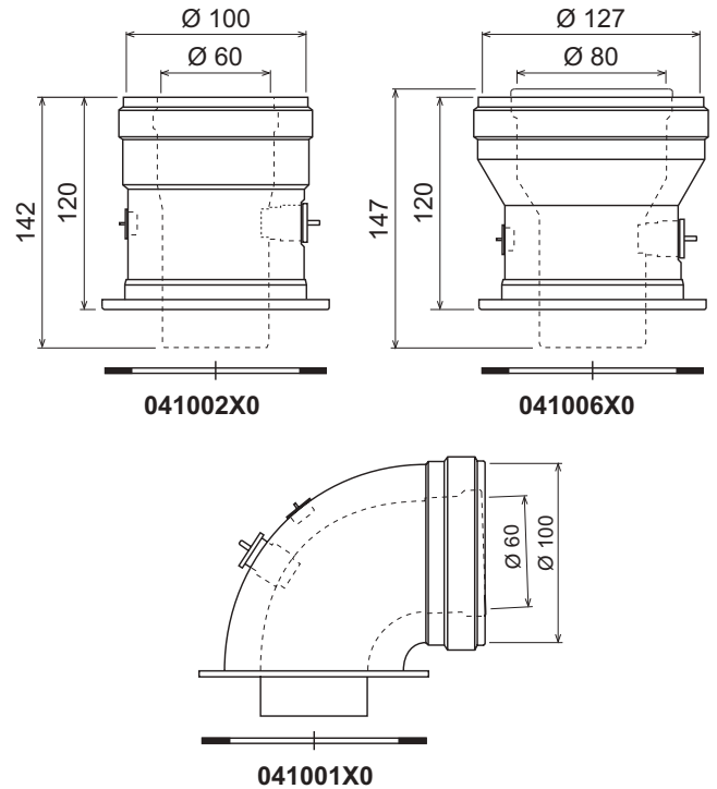
мал. 16 - Початкові елементи для коаксіальних трубопроводів
