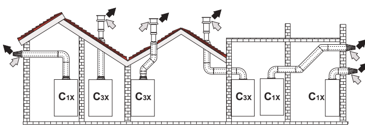
мал. 15 - Приклад підключення за допомогою співвісних (коаксіальних) труб (→ = Повітря / → = Відпрацьовані газів)
