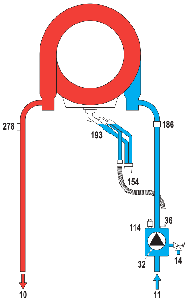
fig. 28 - Circuitul hidraulic
